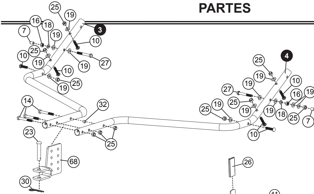
VISTA DEL COMPONENTE DE LA CARCASA DEL CEPILLO:
